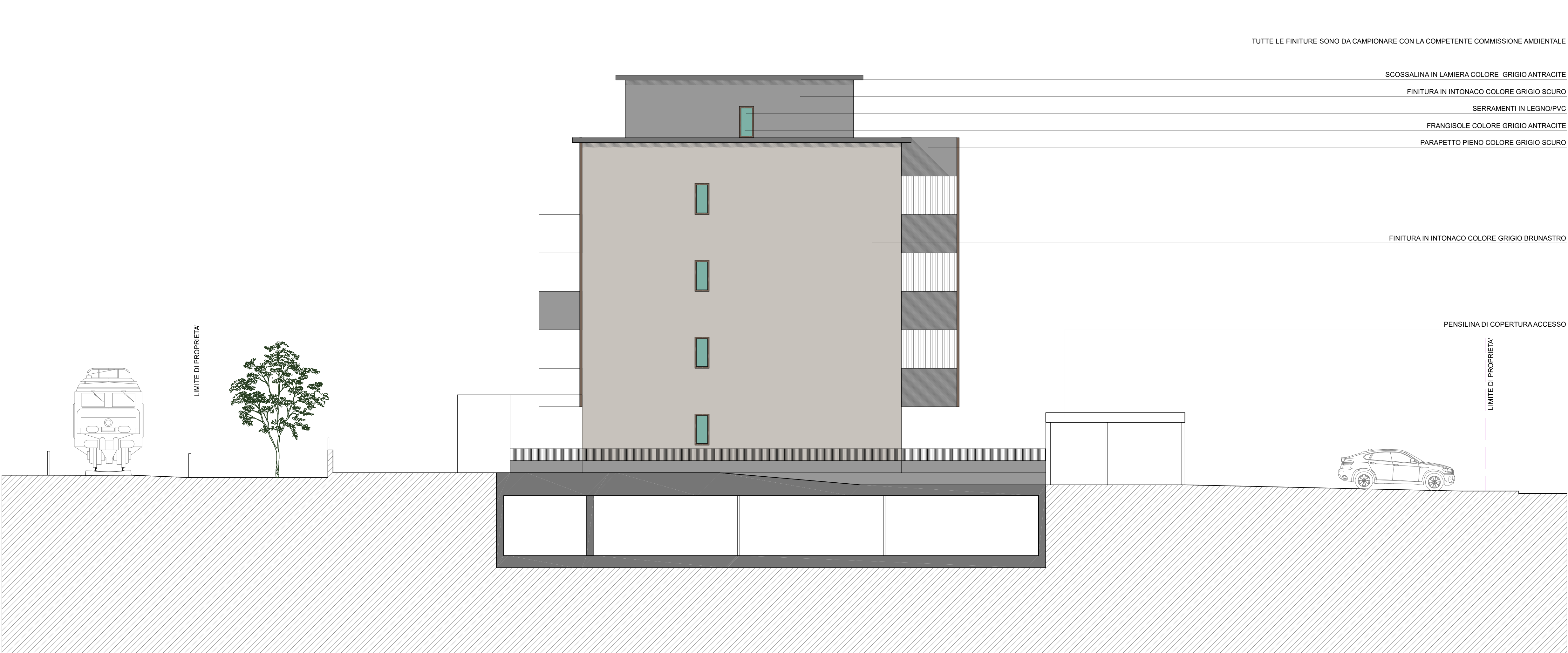
SEZIONE-PROSPETTO G-G
